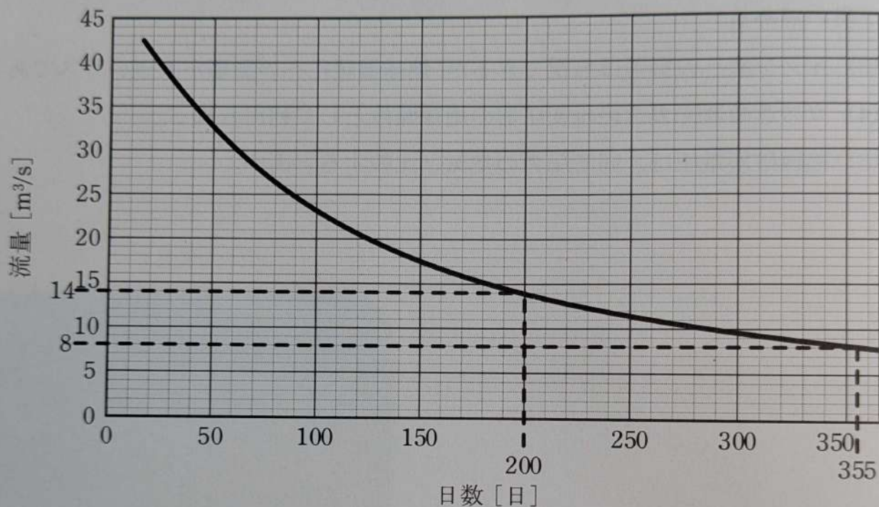
図 流況曲線
